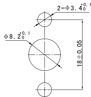
安装开孔尺寸 Mounting hole
