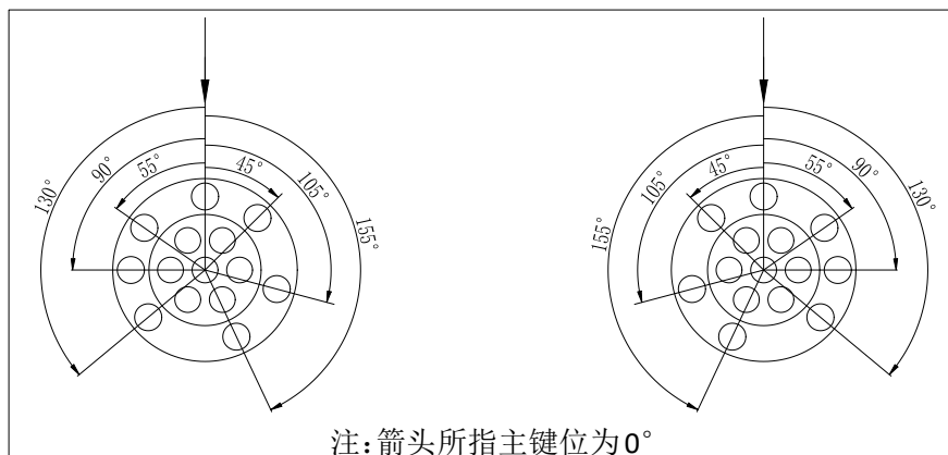
插头插合面视图
