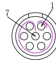
母针芯焊接端 焊接排序图
