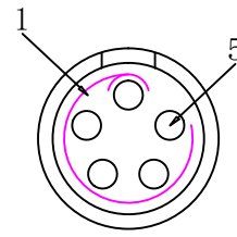
公针芯焊接端 焊接排序图
