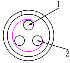
公针芯焊接端 焊接排序图
