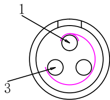
母针芯焊接端 焊接排序图
