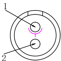
母针芯焊接端 焊接排序图
