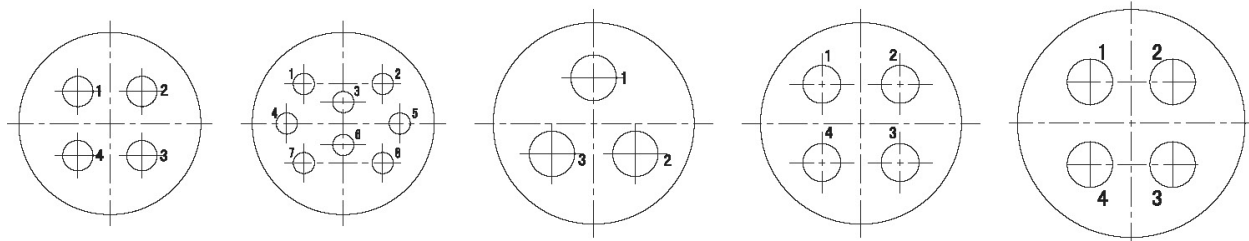
YLD-1804 (4- \phi 4) YLD-1808 (8- \phi 2.5) YLD-2003a (3- \phi 6) YLD-2004 (4- \phi 5) YLD-2204 (4- \phi 6)
