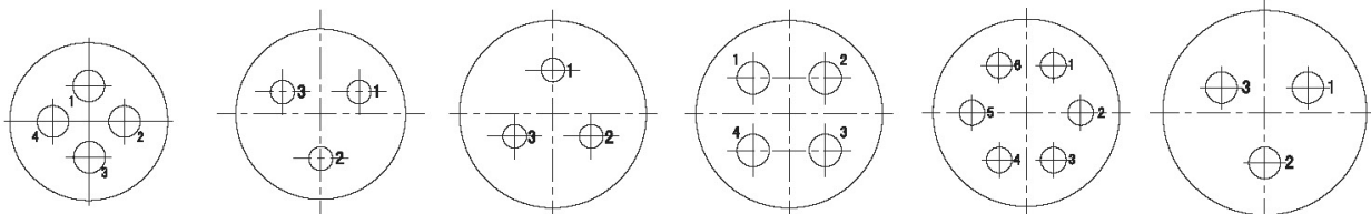
YLD-1404 (4- \phi 3) YLD-1603 (3- \phi 3.5) YLD-1603a (3- \phi 3.5) YLD-1604 (4- \phi 3.5) YLD-1606 (6- \phi 3) YLD-1803 (3- \phi 4)
