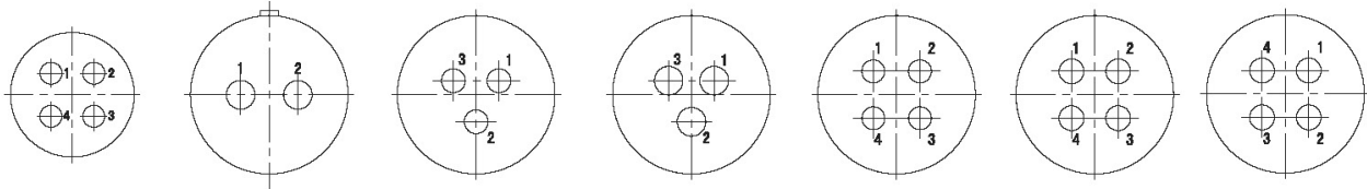
YLD-1004 (4- \phi 1.5) YLD-1202 (2- \phi 2.5) YLD-1203b (3- \phi 2.39) TYLD-1203 (3- \phi 2.5) YLD-1204 (4- \phi 2.2) YLD-1204a (4- \phi 2.39) TYLD-1204b (4- \phi 2.5)
