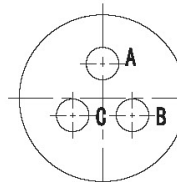
YL-0833 (3- \phi 1.02)
