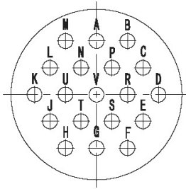
YL-1219 (19- \phi 0.8)
