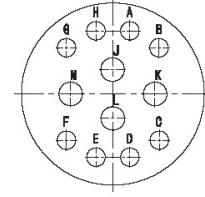
YL-1412a (4- \phi 1.5, 8- \phi 1.02)
