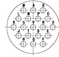
YL-1419 (19- \phi 1.02)
