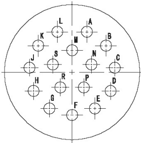
YL-2016 (16- \phi 1.59)
