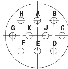
YL-1010a (10- \phi 0.8)
