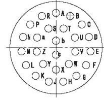
YL-1426 (26- \phi 0.8)
