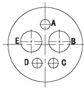
YL-0805 (2- \phi 2, 3- \phi 0.76)
