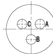
YL-0803 (3- \phi 1.02)
