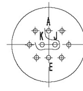
YL-0810 (10- \phi 0.6)
