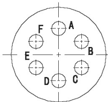
YL-1006 (6- \phi 1.02)
