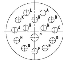
YL-1415 (1- \phi 1.59, 14- \phi 1.02)
