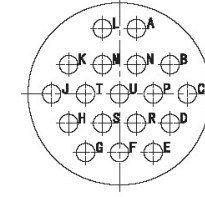
YL-1418 (18- \phi 1.02)
