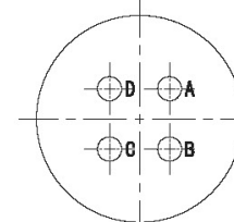
YL-1004 (4- \phi 1.02)
