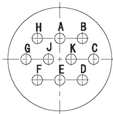
YL-1010 (10- \phi 0.8)
