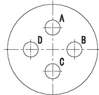
YL-1404a (4- \phi 2.39)
