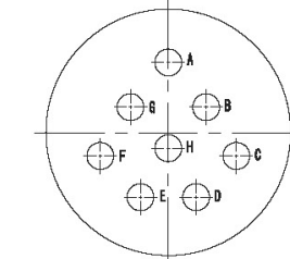
YL-1608 (8- \phi 1.59)
