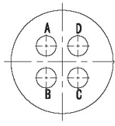
YL-0804b (4- \phi 1.02)
