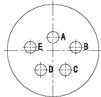
YL-1405 (5- \phi 1.59)
