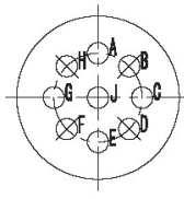
YL-0809 (9- \phi 0.76)
