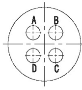
YL-0804 (4- \phi 1.02)
