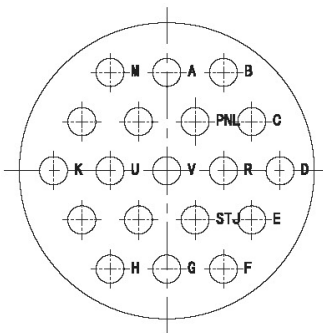
YL-2419 (19- \phi 2.39)
