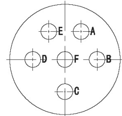
YL-1606a (6- \phi 2.39)
