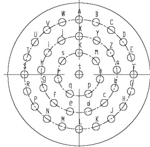
YL-1841 (41- \phi 0.8)
