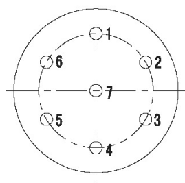
YL-1207 (7- \phi 1.02)
