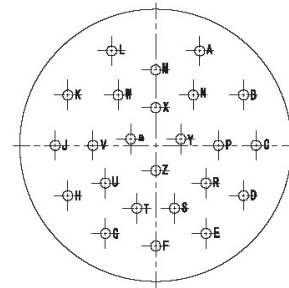
YL-2024 (24- \phi 1.02)
